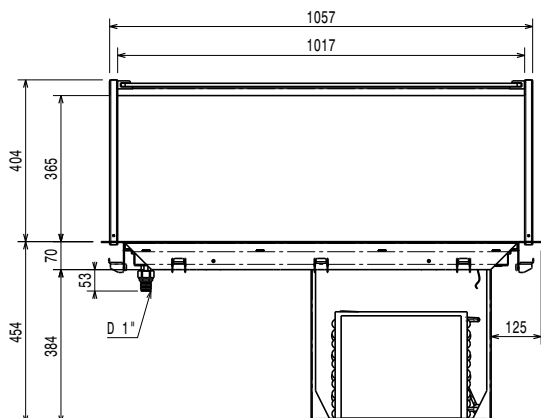
Zepředu
